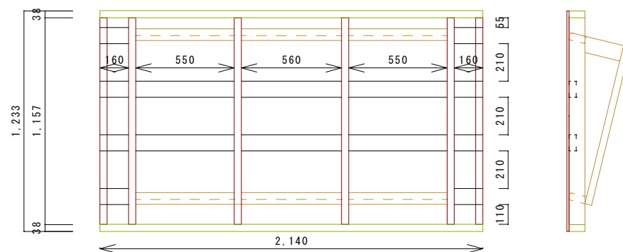
■ 構造材屋根伏せ図
