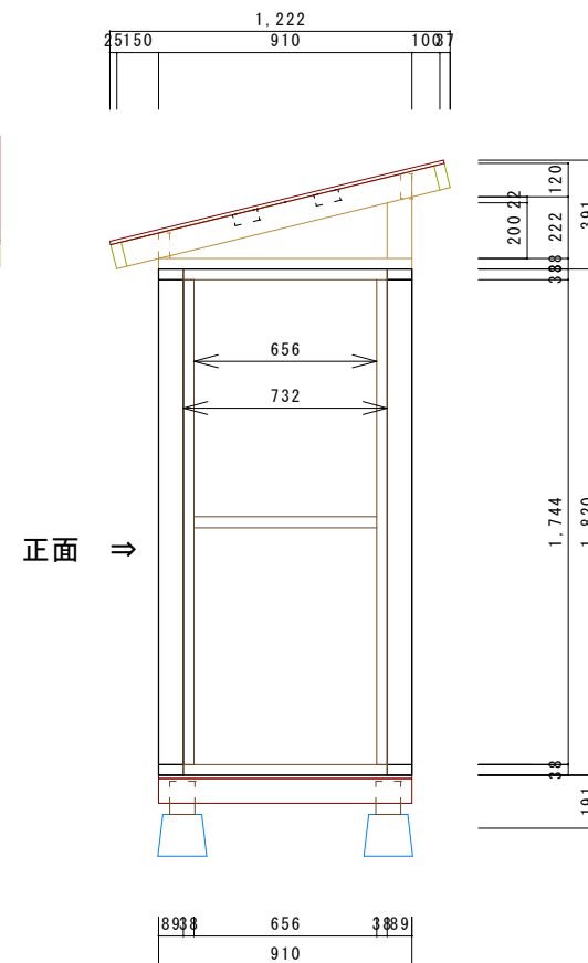
■ 構造材立面図：側面
