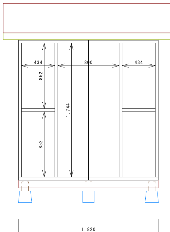
■ 構造材立面図：正面
