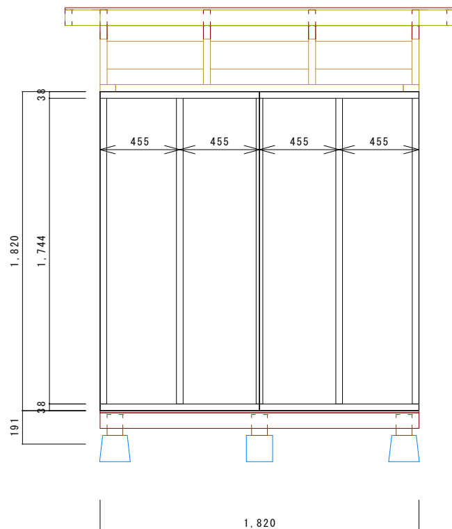
■ 構造材立面図：背面
